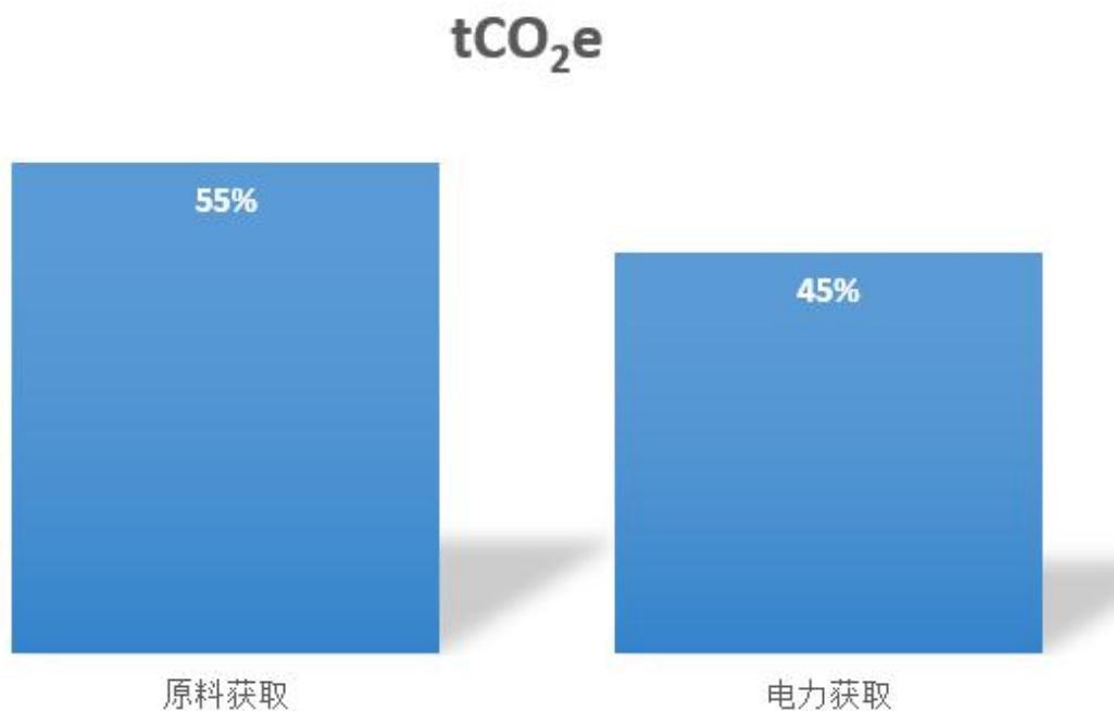
图 4.2 回转窑生命周期各过程碳足迹贡献比例
