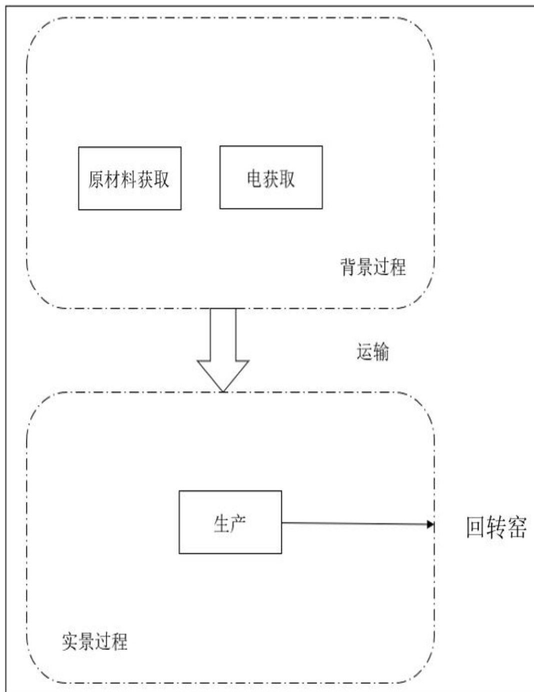
图 2.1 回转窑生产系统边界图
